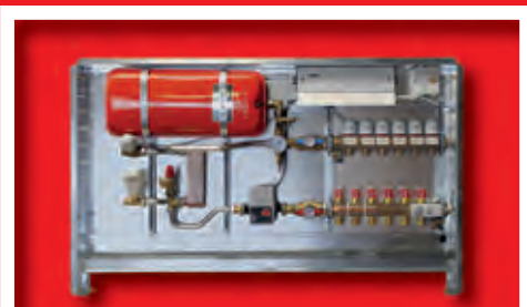
COMPACTFLOOR FWW anschlussfertige Regelstation für Fußbodenheizungen mit Messing-Stangenverteiler
