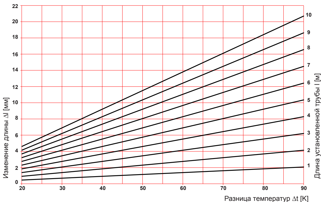
Диаграмма „Тепловое удлинение металлопластиковой композитной трубы PIPEFIX“
