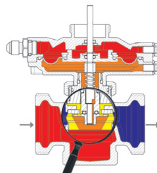
Разгруженный затвор на регуляторе перепада расхода 4001
