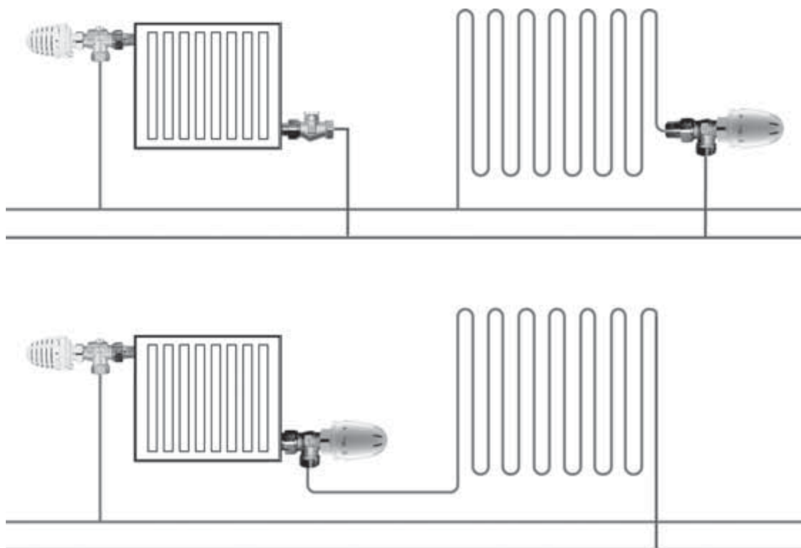
Slika 1 Primer primene regulacije zagrevanja poda u kombinaciji sa radijatorima
