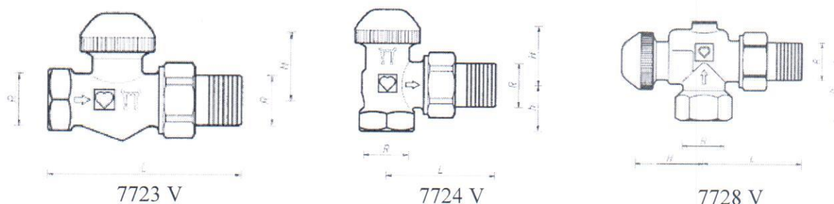
Slika 1. Izgled i dimenzije ventila HERZ-TS-90-V sa skrivenim podešavanjem pravi, ugaoni i ugaoni specijal model
